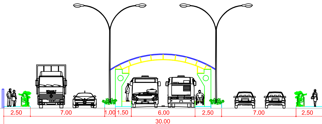
Seção Transversal - Avenida Tronco Alimentadora Gabarito = 30 m
