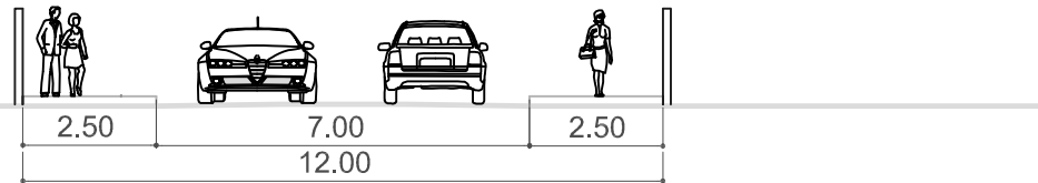
Via Local Gabarito = 12 m
