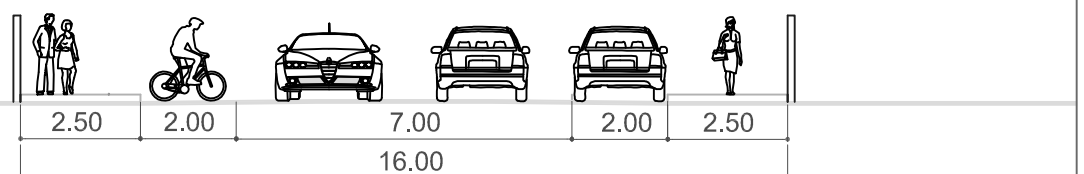
Via Coletora com ciclofaixa unidirecional e estacionamento Gabarito = 16 m
