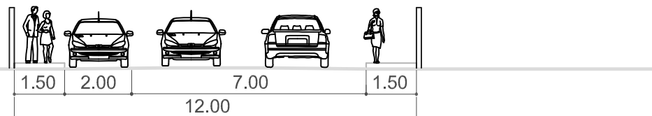
Via Local com estacionamento Gabarito = 12 m
